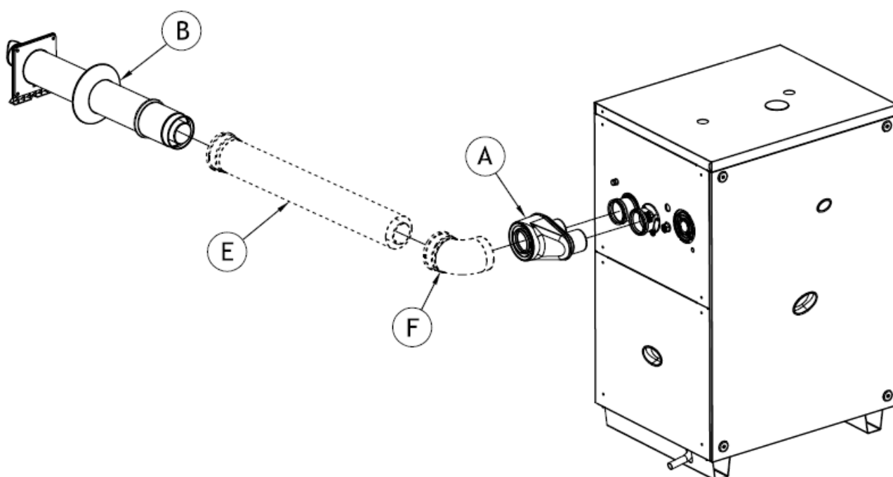
Figura 1 - Installazione tipo C13 - scarico coassiale a parete DN80/125 oppure DN60/100
