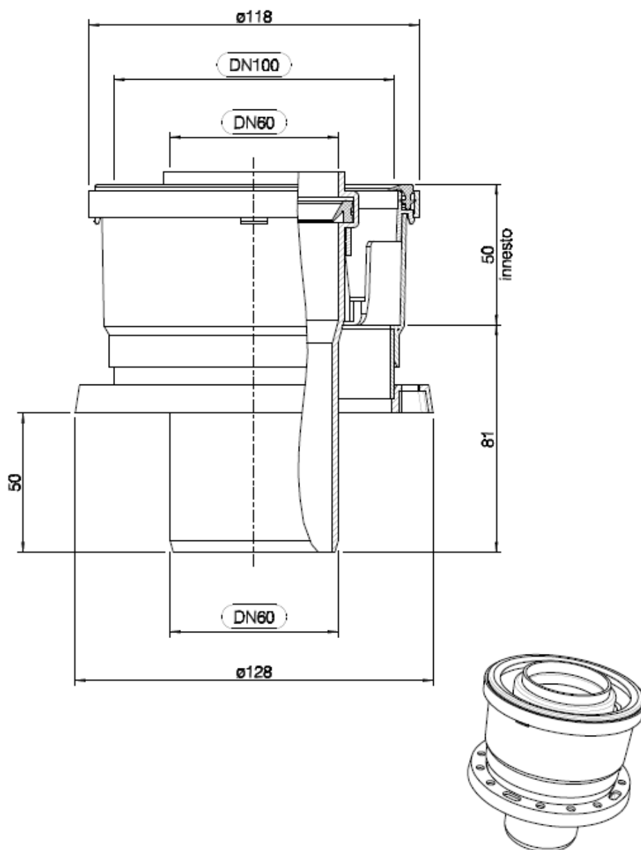
Figura 1 - Esempio adattatore per installazioni AY00-120 tipo C
